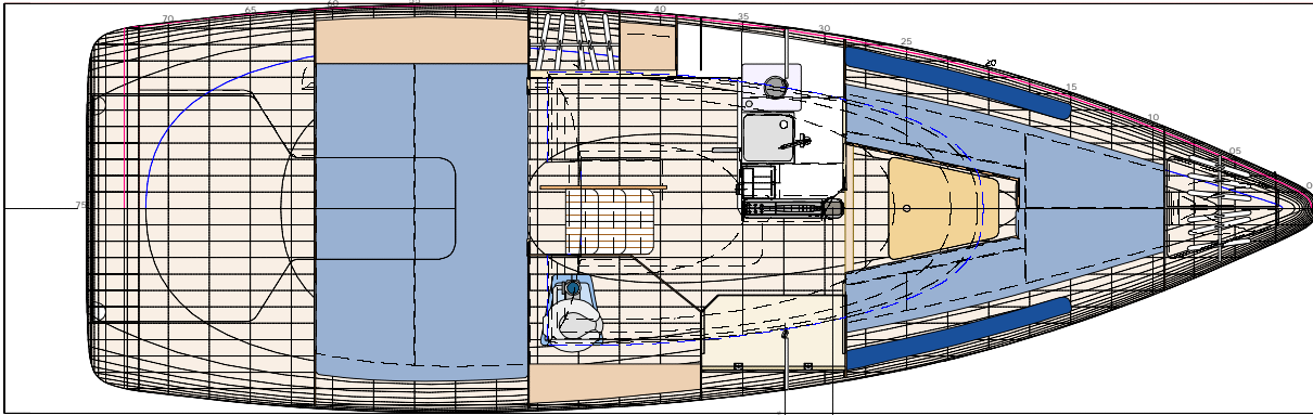
Aménagement - Vue en plan - Echelle 1/10
